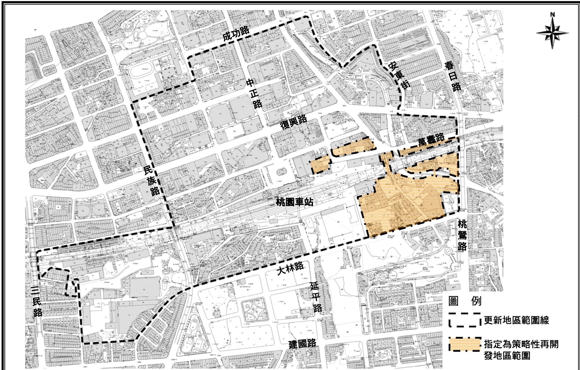
附圖2-2 桃園站區周邊都市更新地區範圍示意圖
